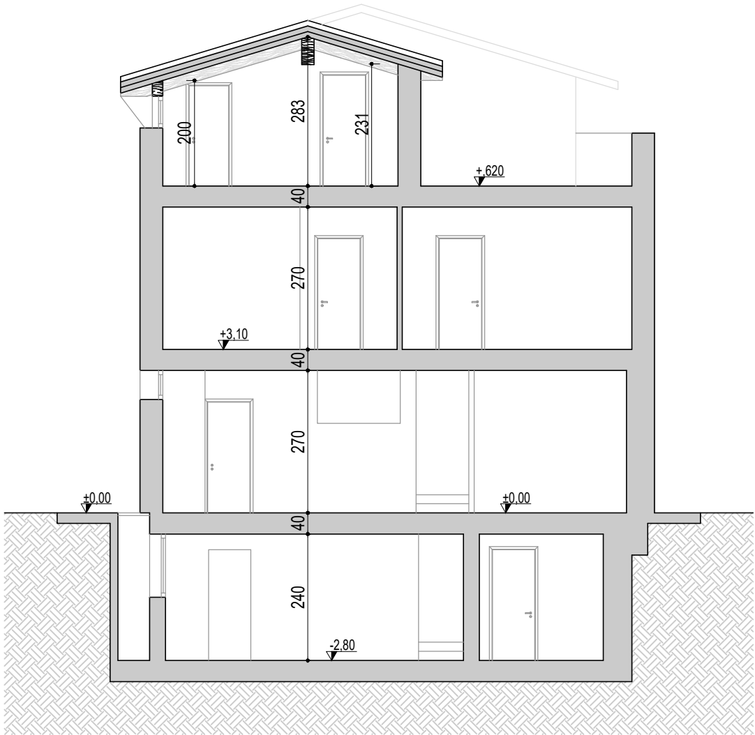
SEZIONE B-B
