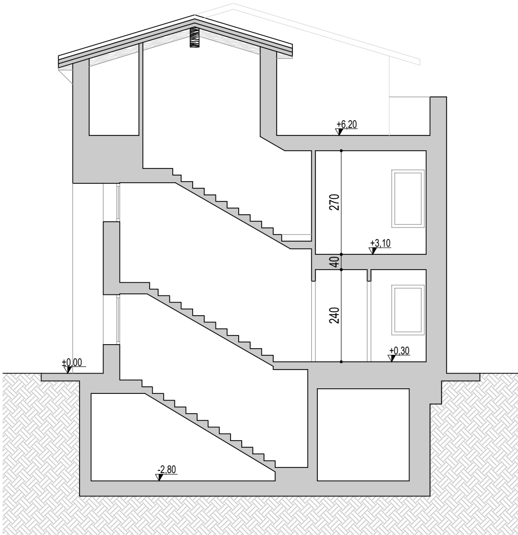
SEZIONE A-A
