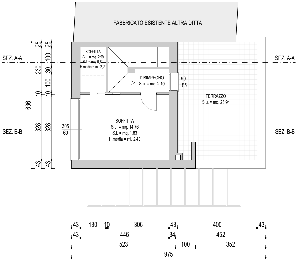
PIANTA PIANO SOTTOTETTO
